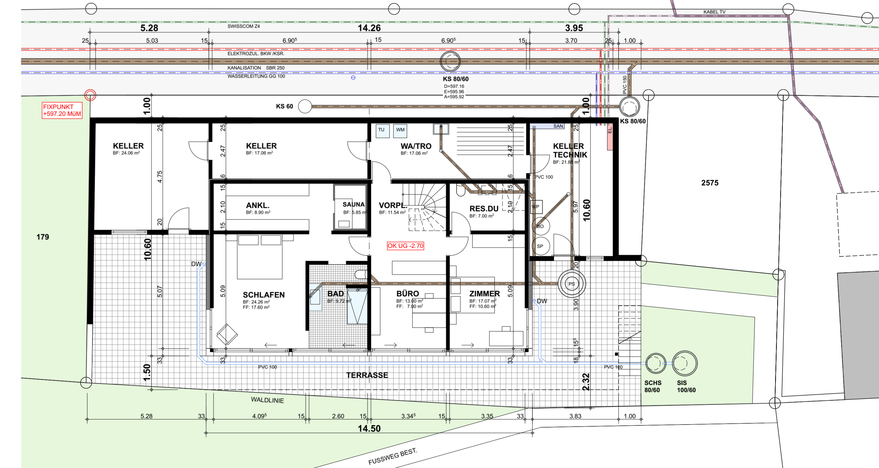
UNTERGESCHOSS
