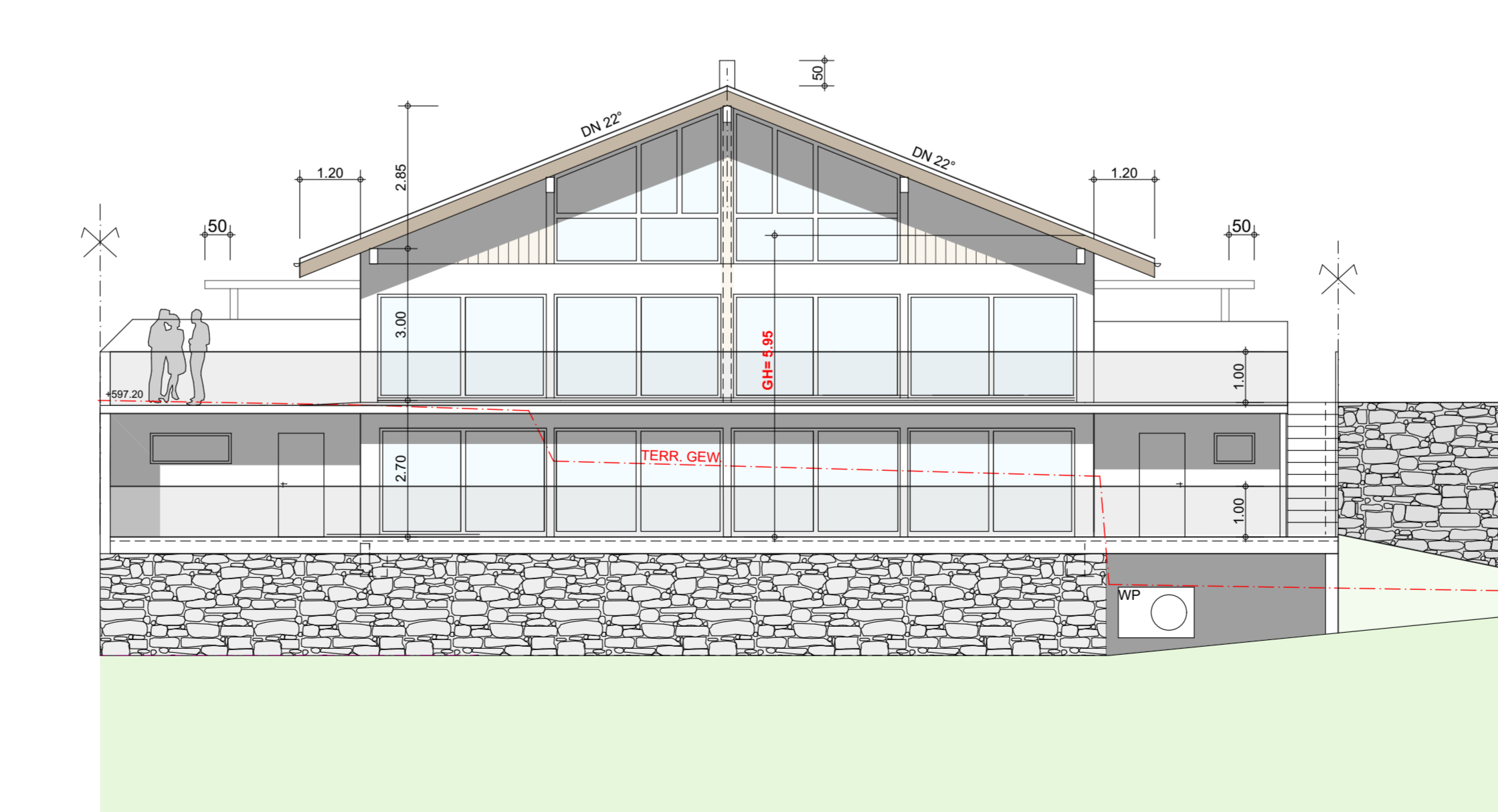
SÜDFASSADE
