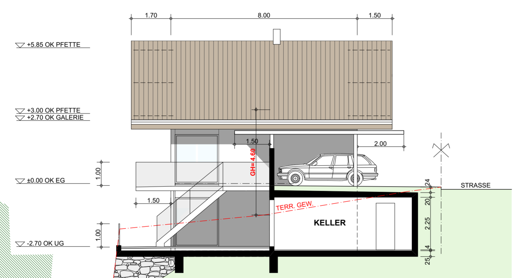
WESTFASSADE
