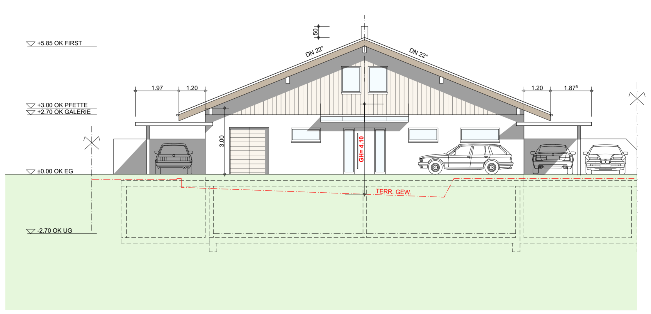
NORDFASSADE
