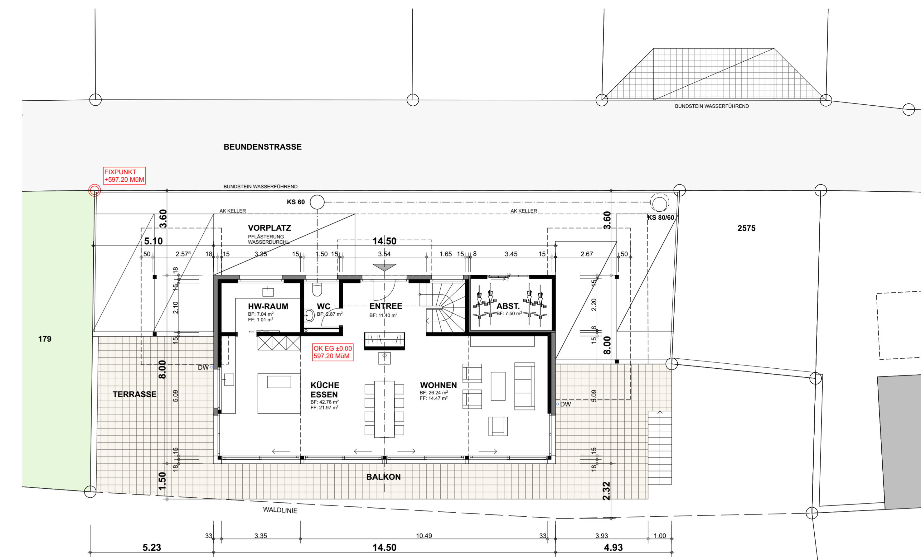
ERDGESCHOSS
