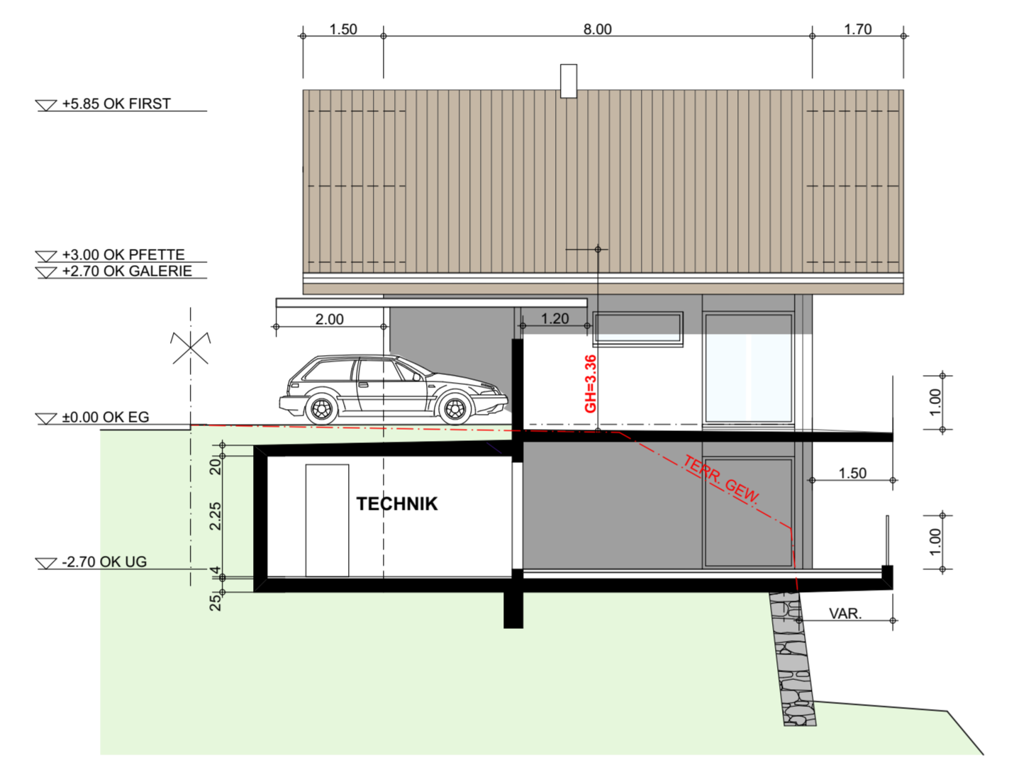
WESTFASSADE
