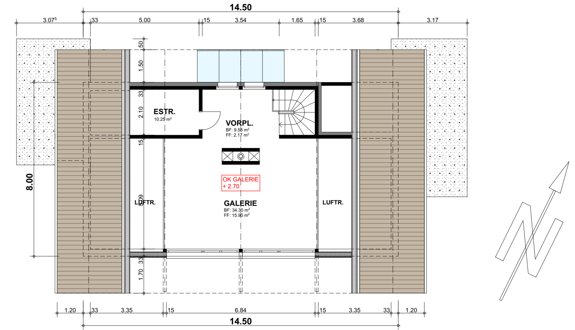
GALERIE
